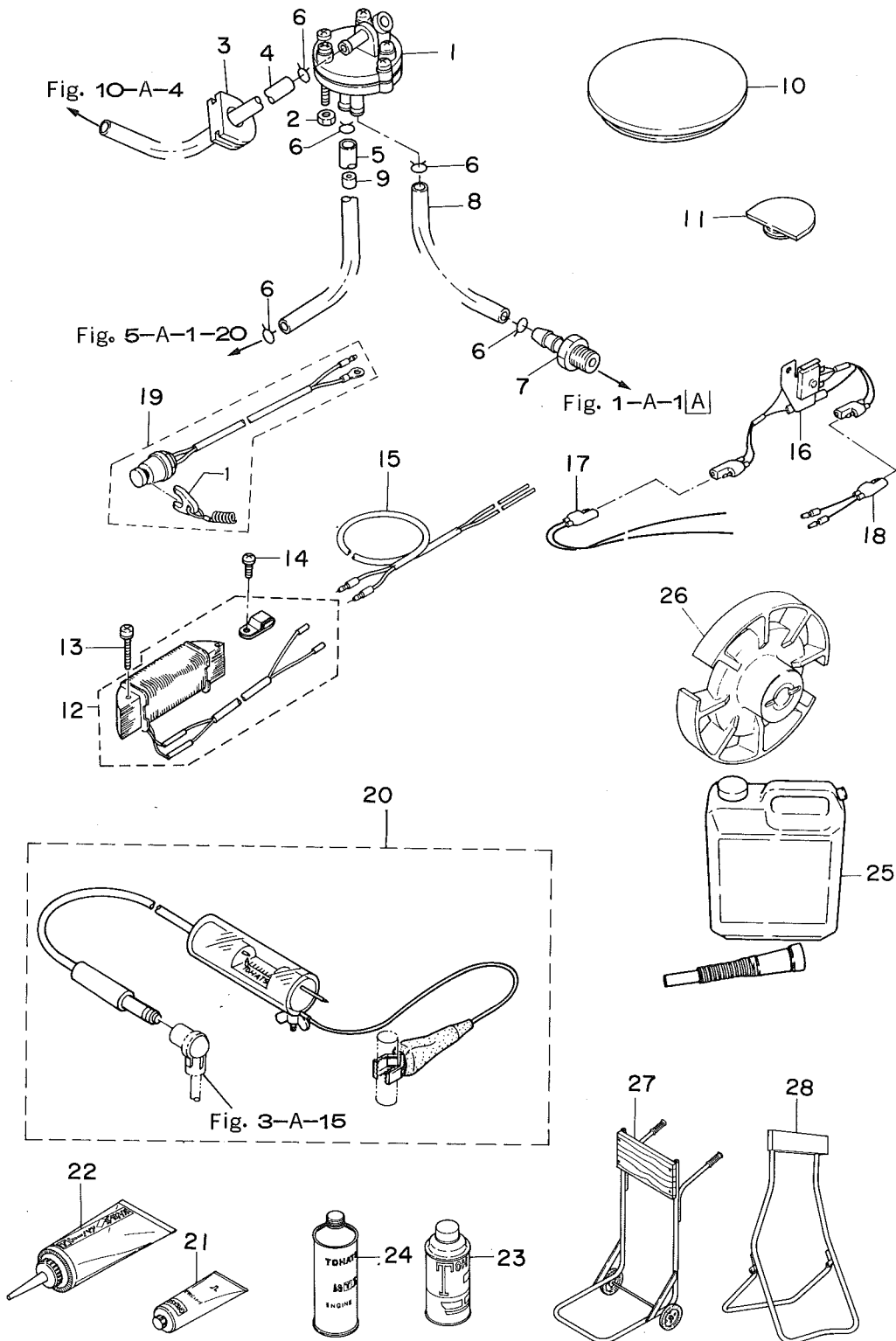
Fig. 12-A OPTIONAL PARTS(3)ACCESSORIES
