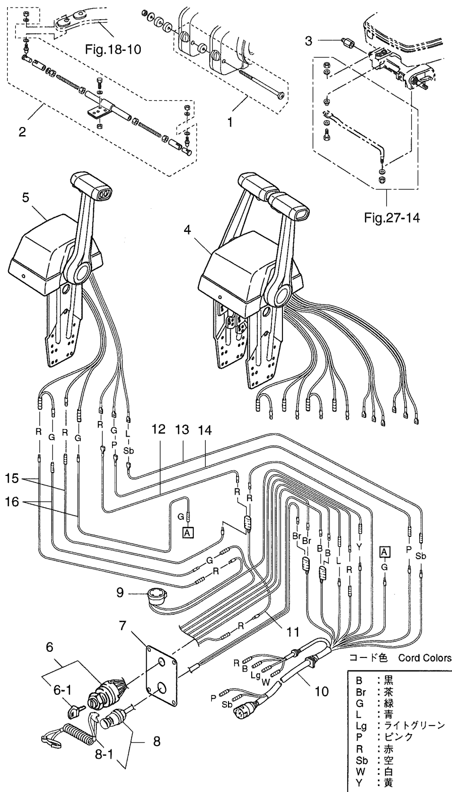
Fig. 29 OPTIONAL PARTS (2)
