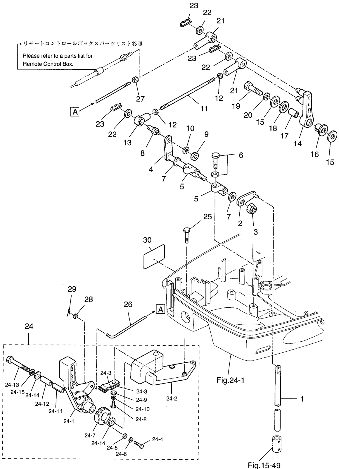
Fig. 17 SHIFT (cont.)
