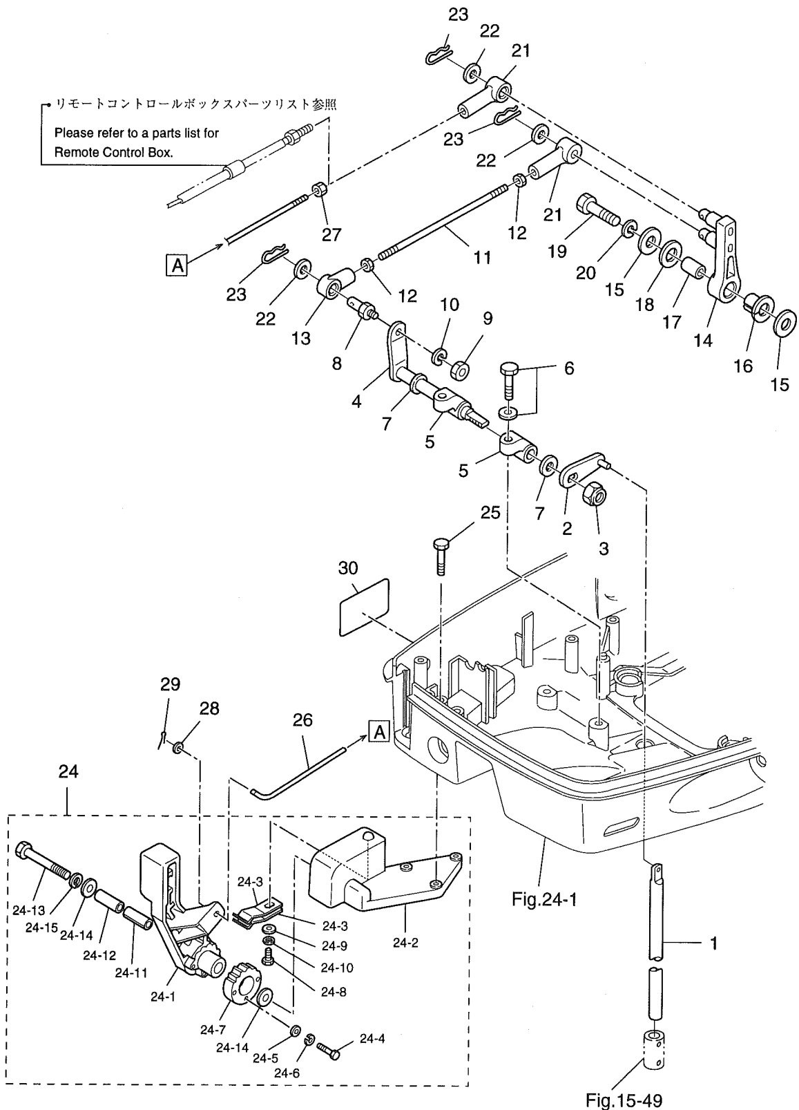
Fig. 17 SHIFT
