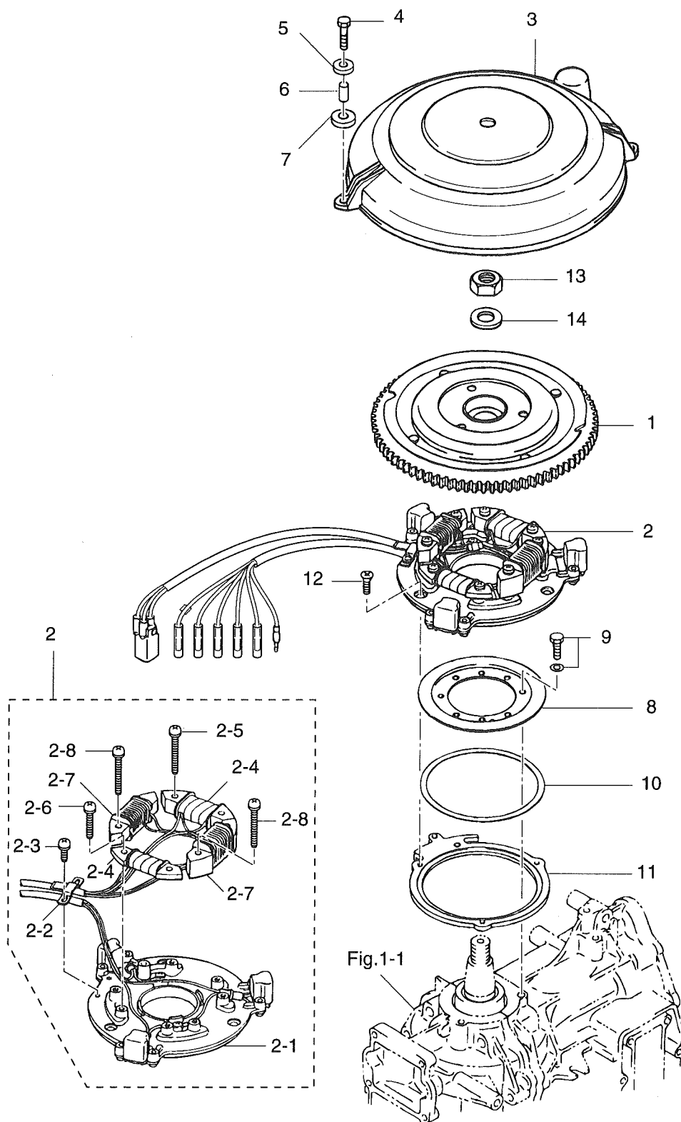
Fig. 9 MAGNETO
