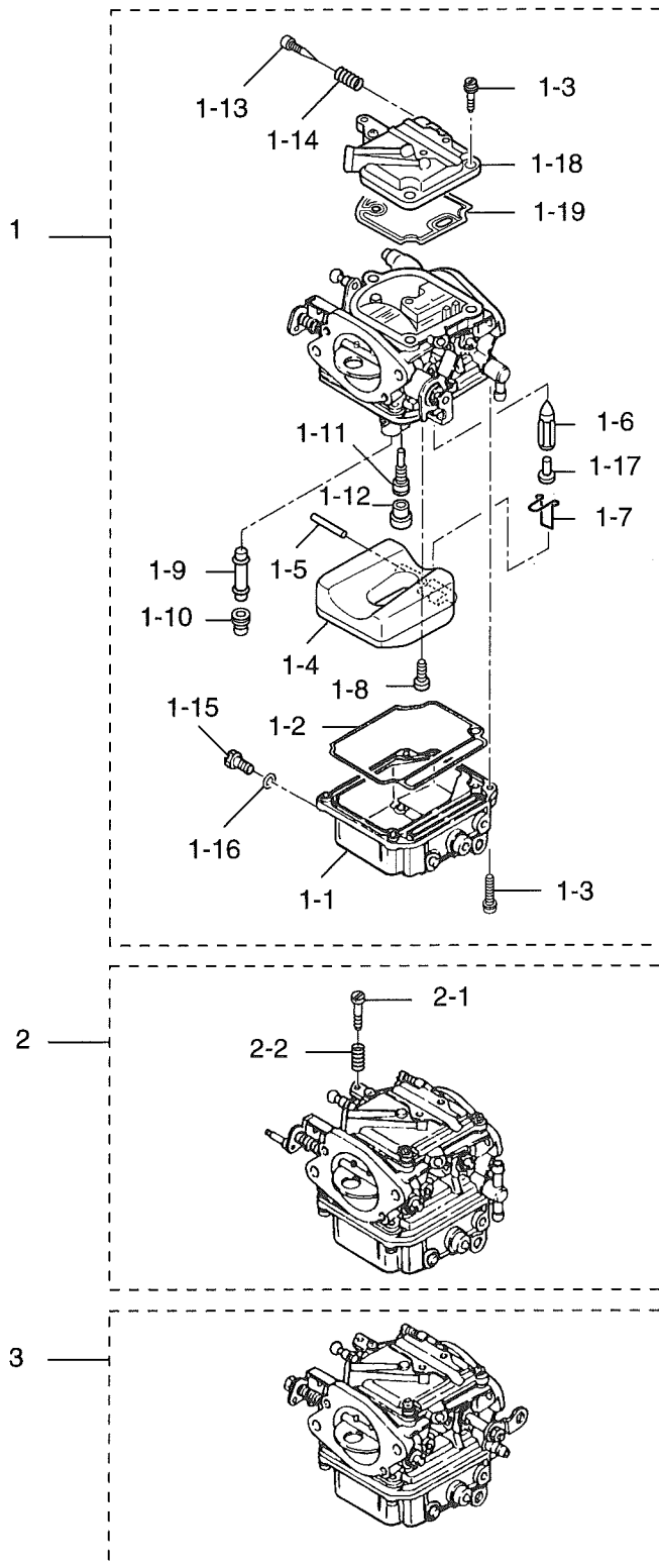
Fig. 5 CARBURETOR
